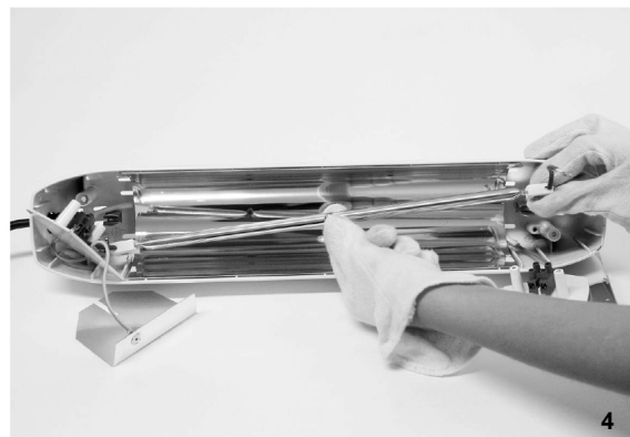
4. ИЗВЛЕКИТЕ ЛАМПУ, ОТСОЕДИНИВ ЕЕ ОТ ПРУЖИН. ВСТАВЬТЕ НОВУЮ ЛАМПУ В ПРУЖИНЫ, ТАКИМ ОБРАЗОМ, ЧТОБЫ ПРЕДВАРИТЕЛЬНО УКРОЧЕННЫЕ ПРОВОДА ЛАМПЫ БЫЛИ ВТАВЛЕНЫ В ЗАЖИМЫ. СОБИРИТЕ ЗАНОВО ОБОРУДОВАНИЕ, ПОВТОРИВ ВЫШЕ ПЕРЕЧИСЛЕННЫЕ ОПЕРАЦИИ В ОБРАТНОМ ПОРЯДКЕ ОТ ОПИСАННОГО.
